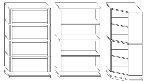
Tiefe 280 mm Korpuselemente 28 Höhe je Element 339/678 mm
