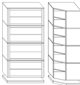
Tiefe 347 mm Korpuselemente 34 Höhe je Element 419 mm
